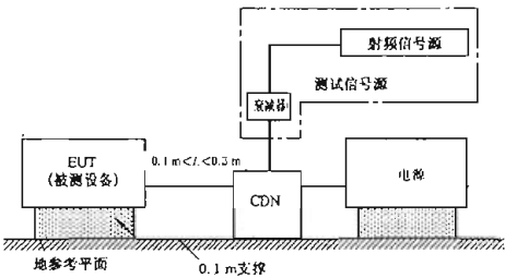
布置图
